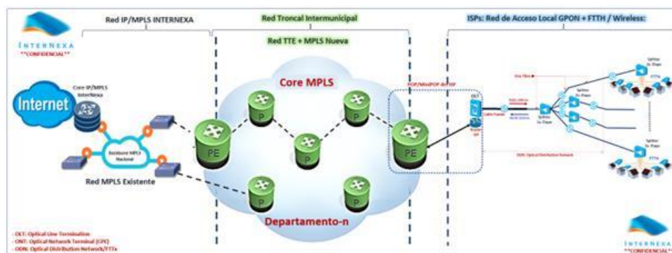
Gráfico 1. Arquitectura de Red Internexa
